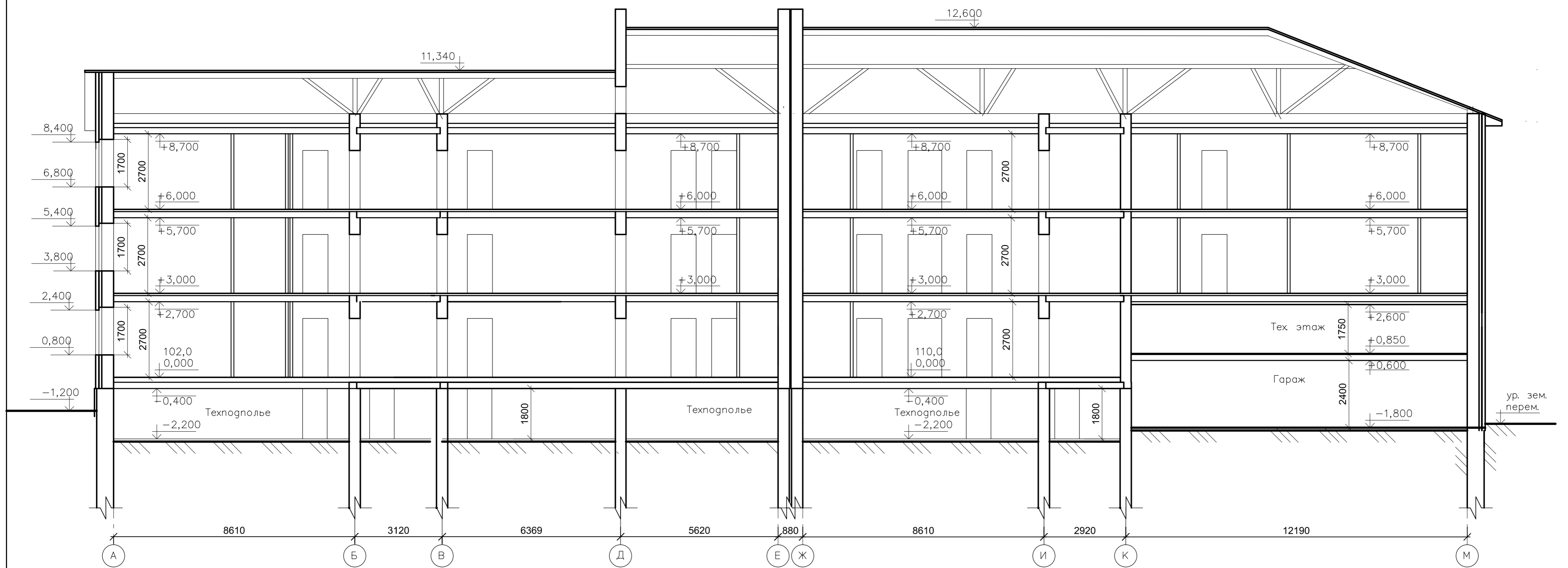
Разрез 2-2, М 1:100.
